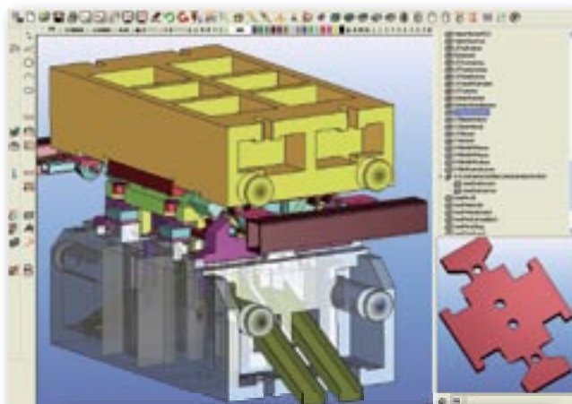
Darstellung der Einzelteile eines Folgeverbundwerkzeuges im grafischen Konstruktionsmanager von MegaCAD
